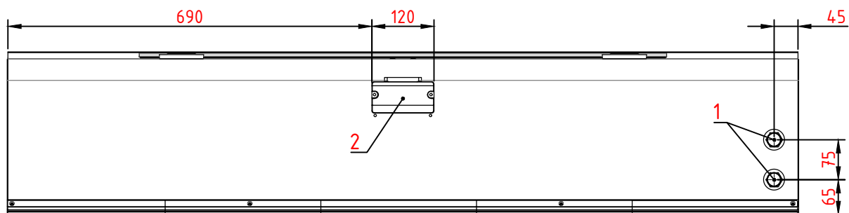
Вид спереди
