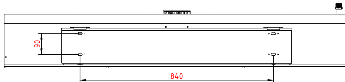
Вид сзади
