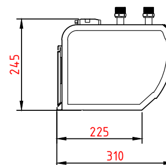
Вид сбоку
