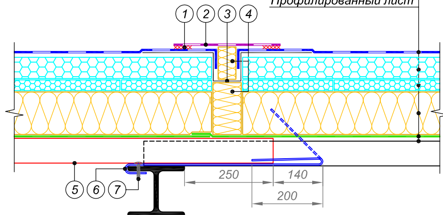
Деталь 3
