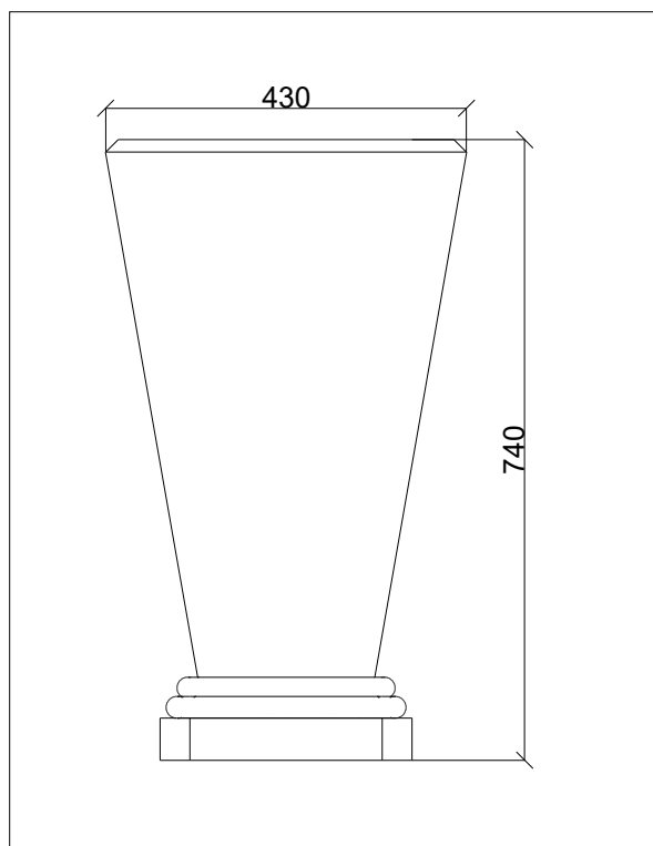
Side/Front (M1:10)
