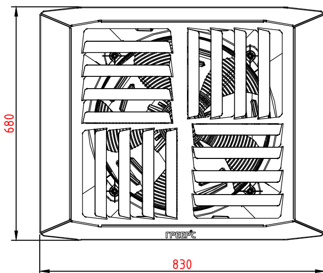
Вид сзади
