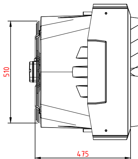
Вид сверху
